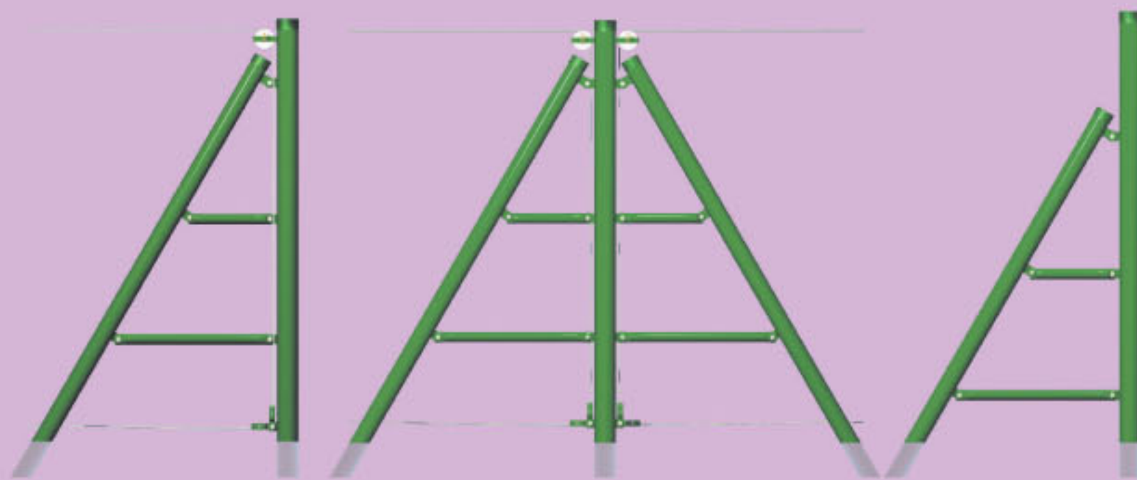
POTEAU DE DÉPART + JAMBE DE FORCE
