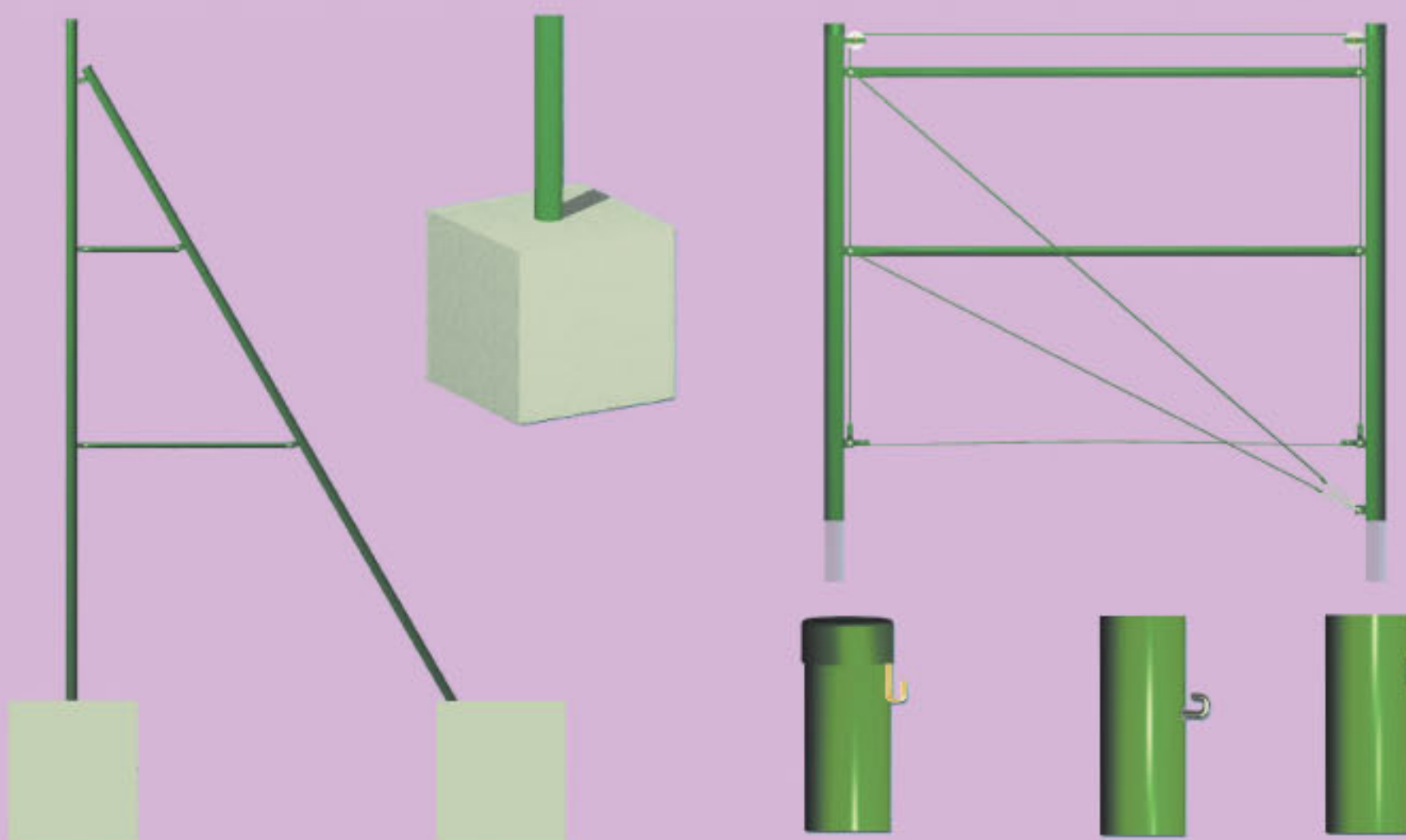
POTEAU INTERMÉDIAIRE + CONTREVENTEMENT 2 ENTRETOISES AU DELÀ DE 8m Hs.
